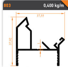
803 0,400 kg/m 45° Dönüş Profili 45° Return Profile
