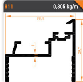
811 0,305 kg/m Sabit Cam Kilit Karşılığı Profili Constant Glass Lockroom Profile
