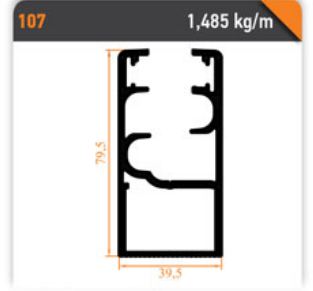
Büyük Düz Kasa Profili Big Straight Case Profile
