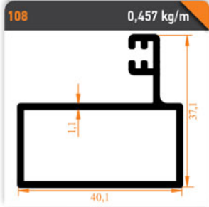
Geniş Yan Dikme Wide Side Pillar
