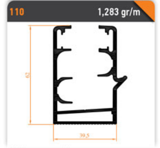
Oluklu Kasa Profili Straight Case Profile
