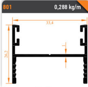
801 0,288 kg/m Isıcam Düz Kapak Profil Double Glazing Straight Cap Profile
