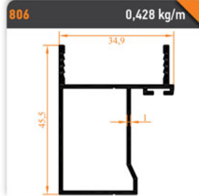
806 0,428 kg/m 90° Dönüş Profili 90° Return Profile
