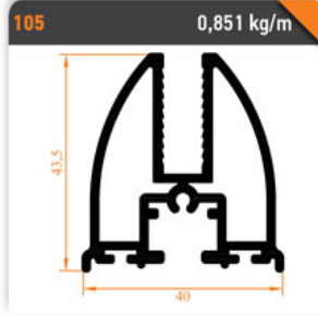
Fırtına Baza FIRTINA Base
